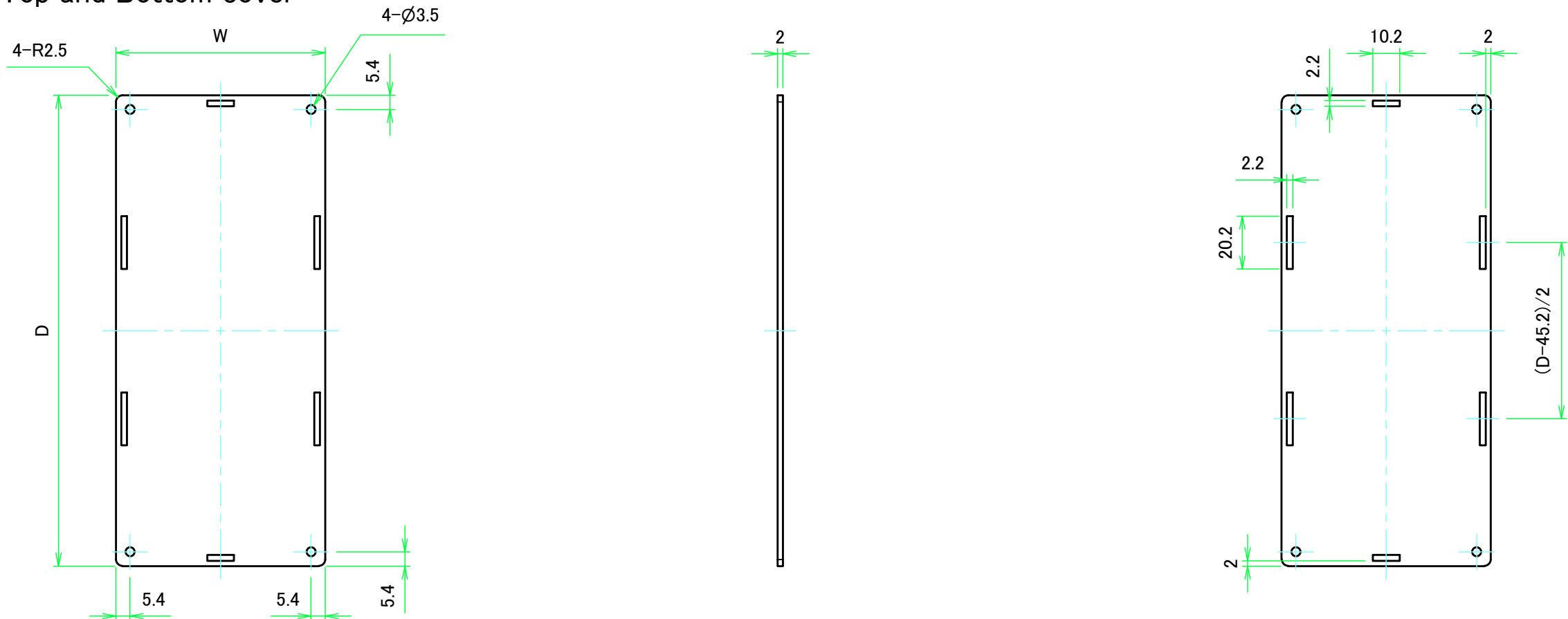
上カバー表面 / Top cover Frontside
