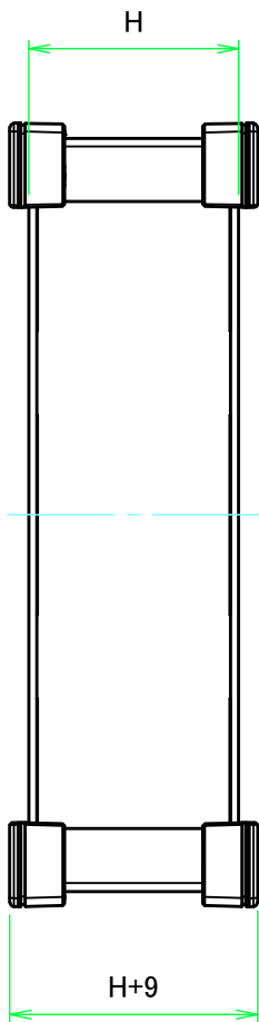
Dパネル2 / D Panel 2
