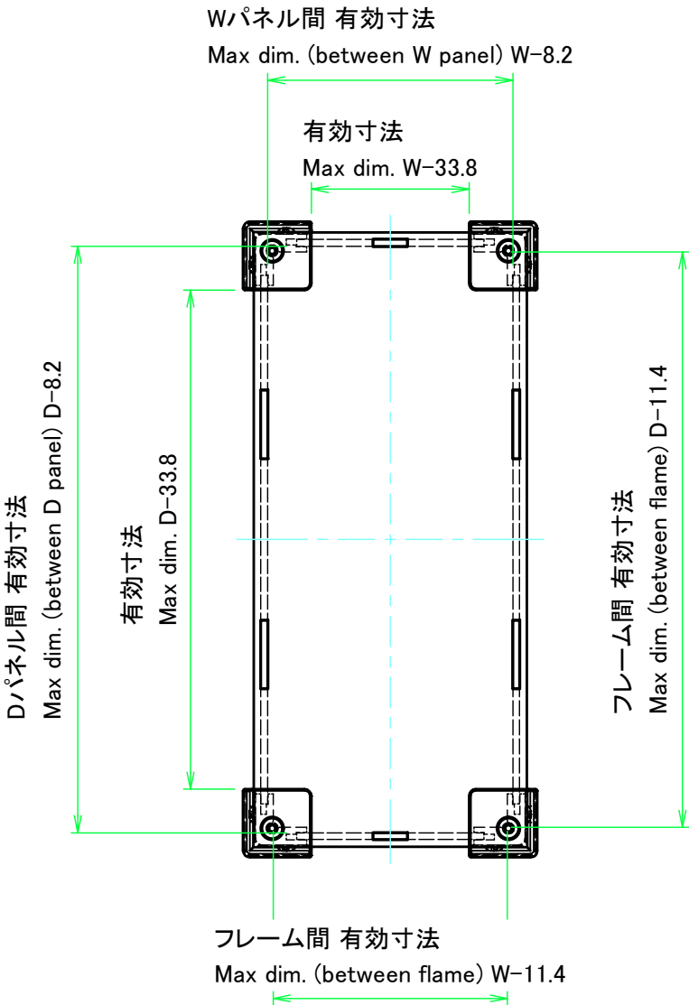
下カバー / Bottom cover
