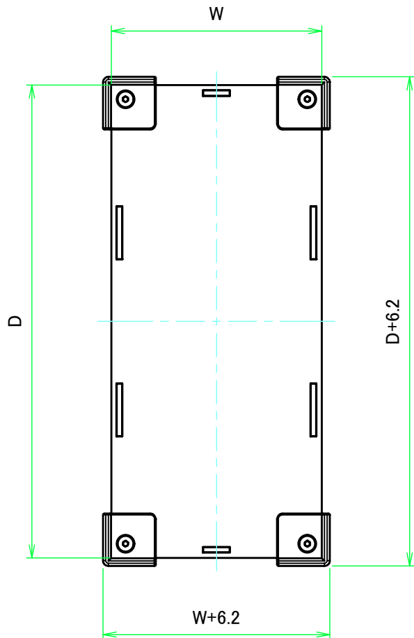
Wパネル1 / W Panel 1
